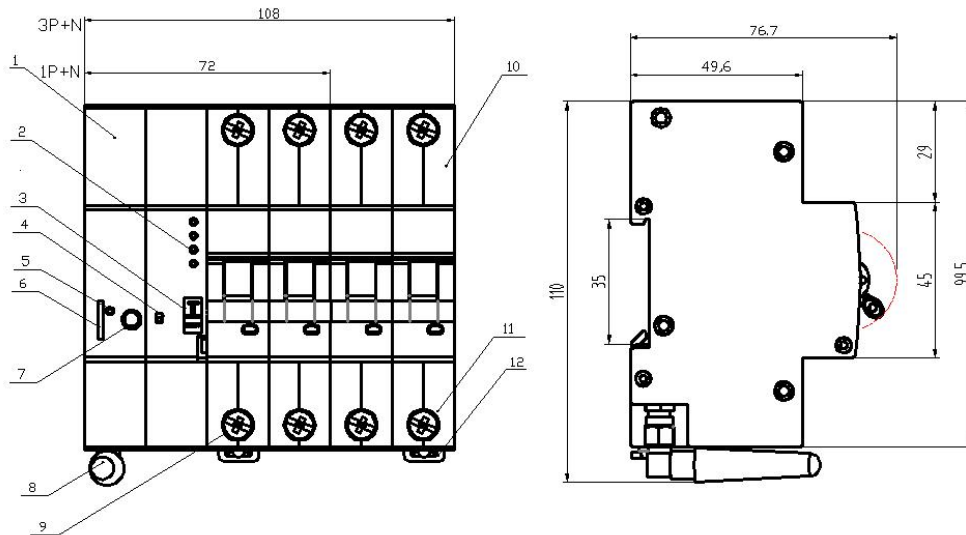
JL1B5LEU-63M(100M) 外形与安装尺寸图
